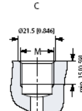
C: G ports (P, T, L, R) M: DIN 3852-2 - G ¼
