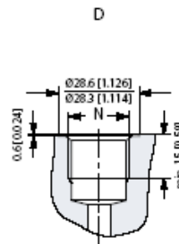
D: G ports w. spot face (P, T, L, R) N: DIN 3852-2 - G ¼
