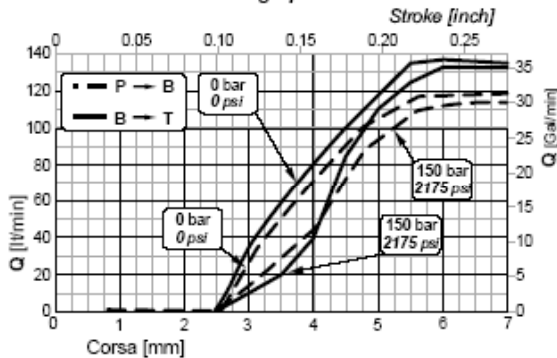
Curve di progressività Metering spool
